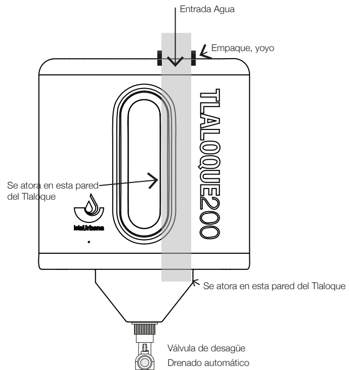
VISTA FRONTAL CORTE
